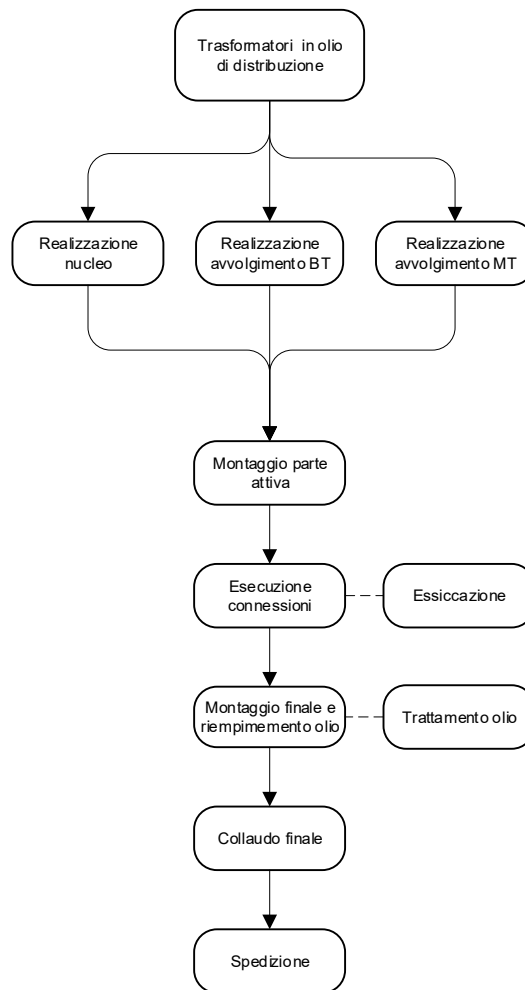
Figura 1 - Processo produttivo del trasformatore TTO ECO+P 400 kVA 20/8,40 - 0,42/0,242 kV
