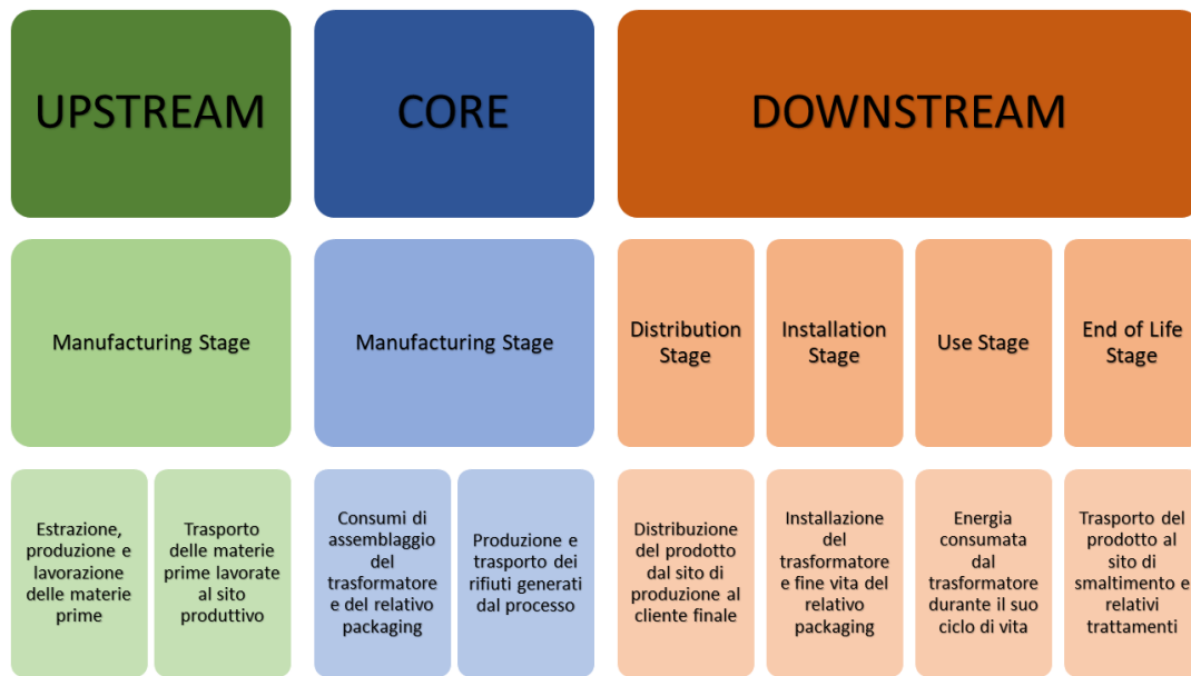
Figura 2 - Confini di sistema di TTO ECO+P 400 KVA 20/8,40 - 0,42/0,242 KV.
