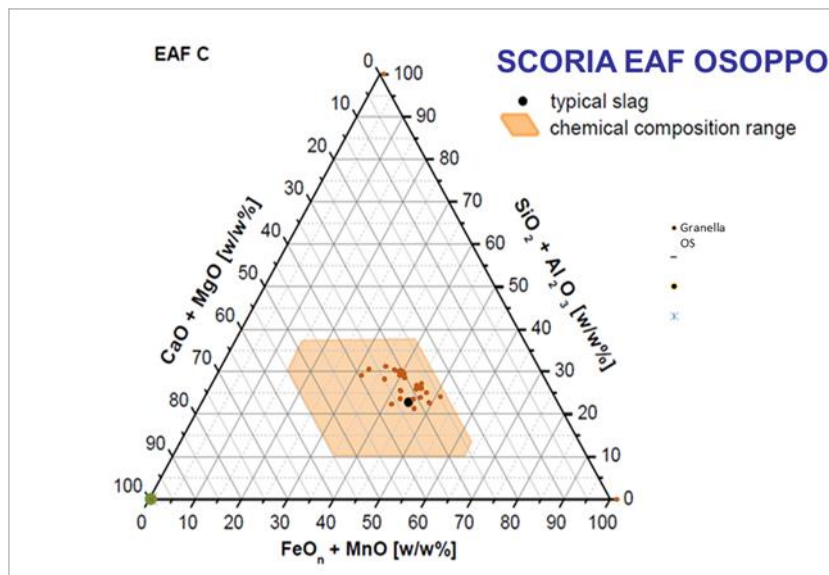
Figura 1 – Diagramma ternario relativo alla scoria prodotta dallo stabilimento di Osoppo. I punti rappresentano le singole analisi effettuate nel corso del 2020.
