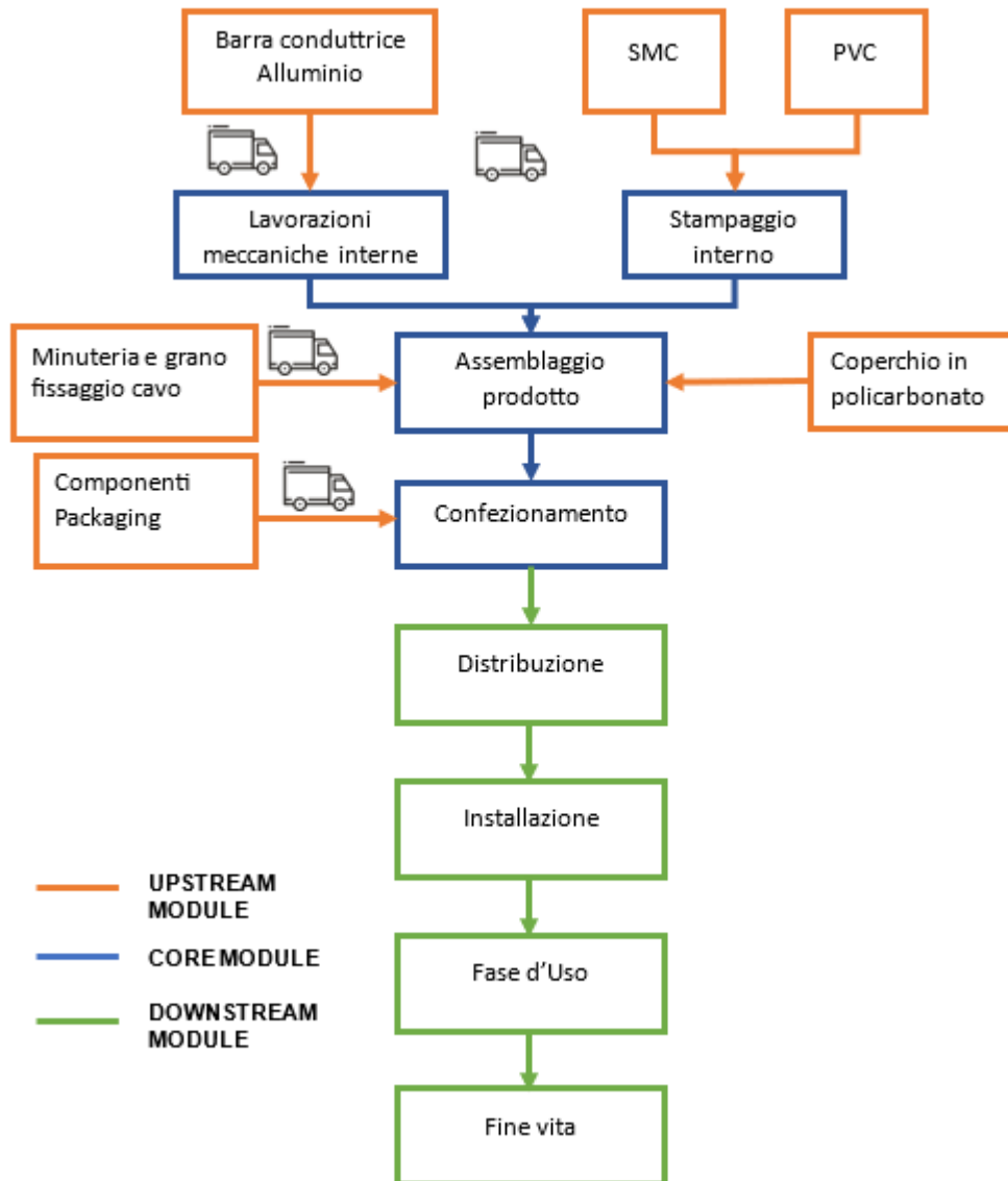
Fig. 1 Flow chart produzione interna della morsettieria
