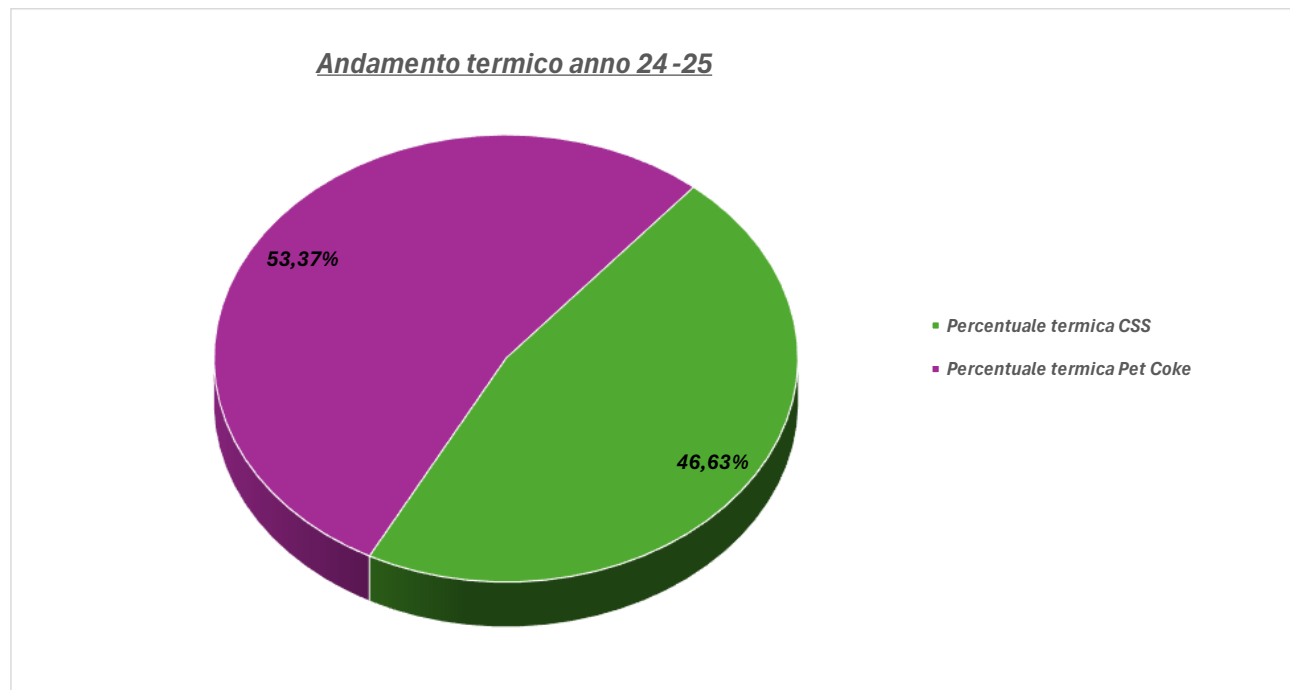
Figura 3 – % sostituzione termica periodo di riferimento.
