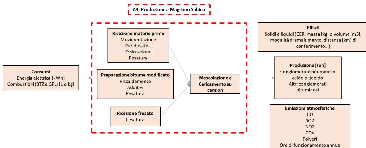
Figura 2: Schema della produzione di un conglomerato bituminoso tiepido prodotto da AMPLIA Infrastructures S.p.A.
