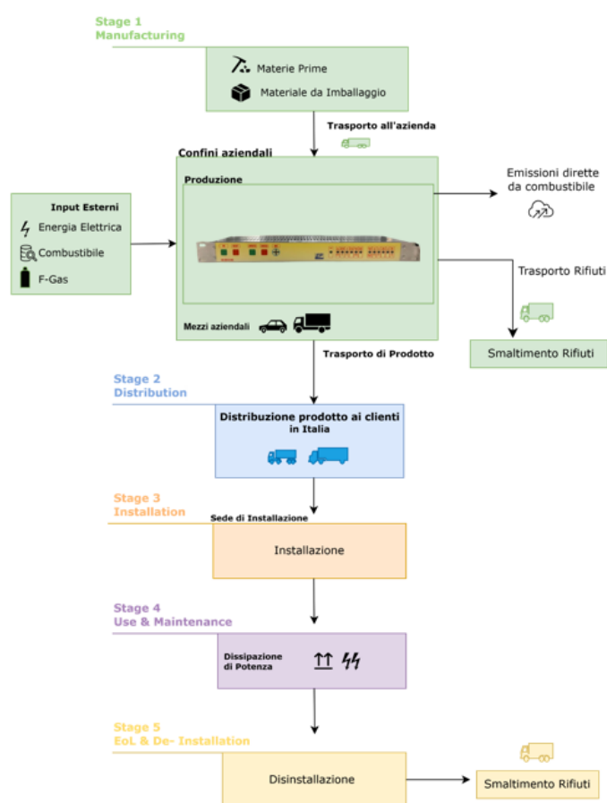
Figura 3 - Diagramma di flusso che schematizza il processo produttivo del "Dispositivo di comando e controllo interruttore di manovra sezionatore ibrido (DQ2026A2NCI)"
