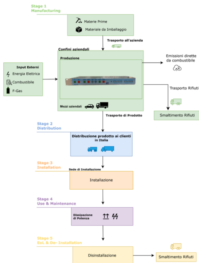
Figura 3 - Diagramma di flusso che schematizza il processo produttivo del "Dispositivo di comando e controllo interruttore di manovra sezionatore (DQ1987A2NCI)"
