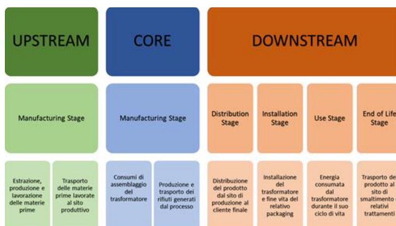
Figura 3 - Confini di sistema di OTN ECO+P 16 MVA 30-15,6 kV.
