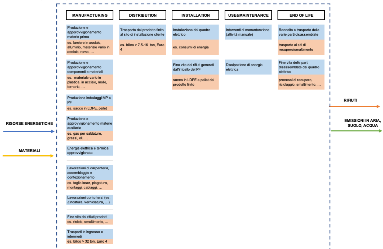
Figura 1: Confini del sistema LCA - EN 50693:2019
