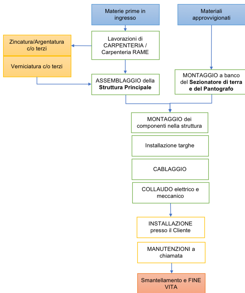
Figura 2: diagramma del processo produttivo del quadro elettrico di tipo "Compatto"
